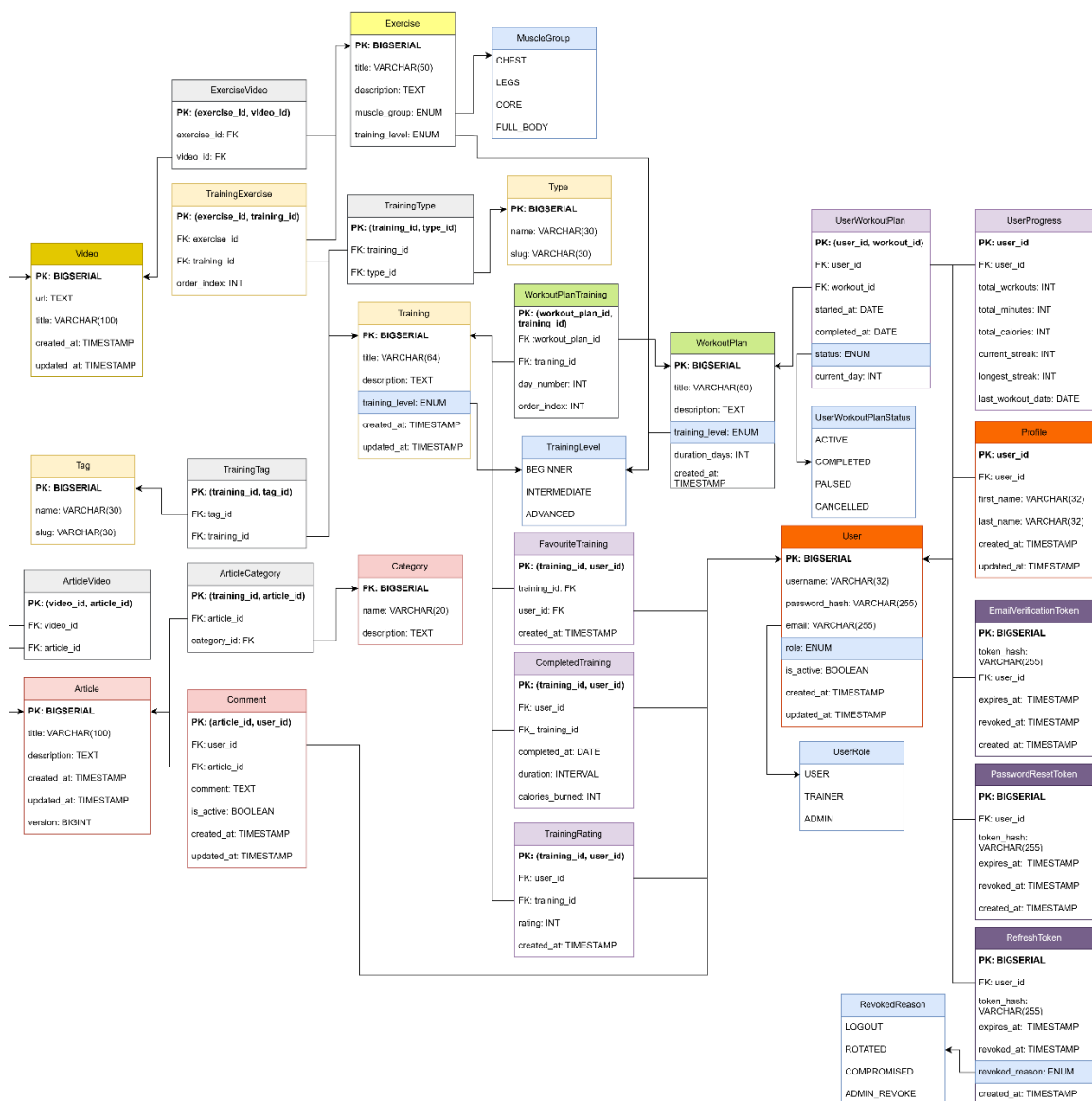
Рисунок 1 – Нотация ERD
